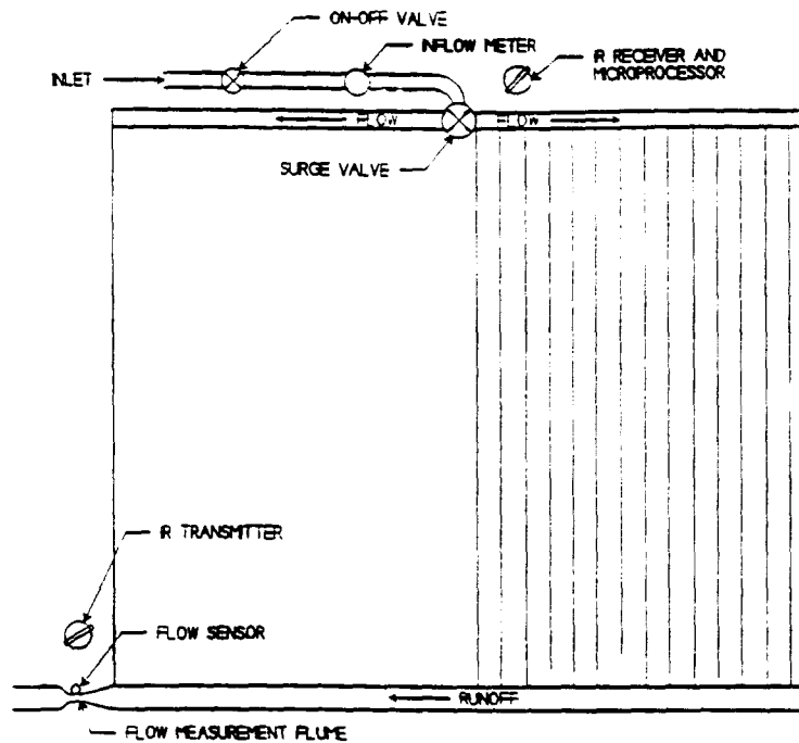
Figure 1. Schematic diagram of a surge feedback control system. (Diagramme schématique d'un système de contrôle d'irrigation à impulsions.)
