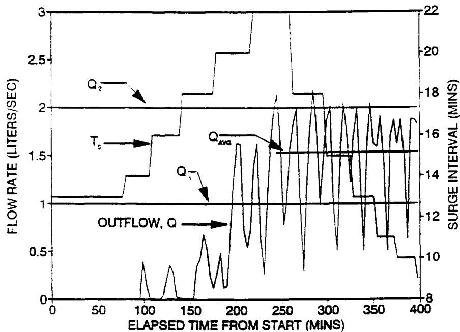
Figure 3. Output diagram for a bean field with a low infiltration rate. (Diagramme des résultats pour un champ d'haricot avec un taux d'infiltration faible.)
