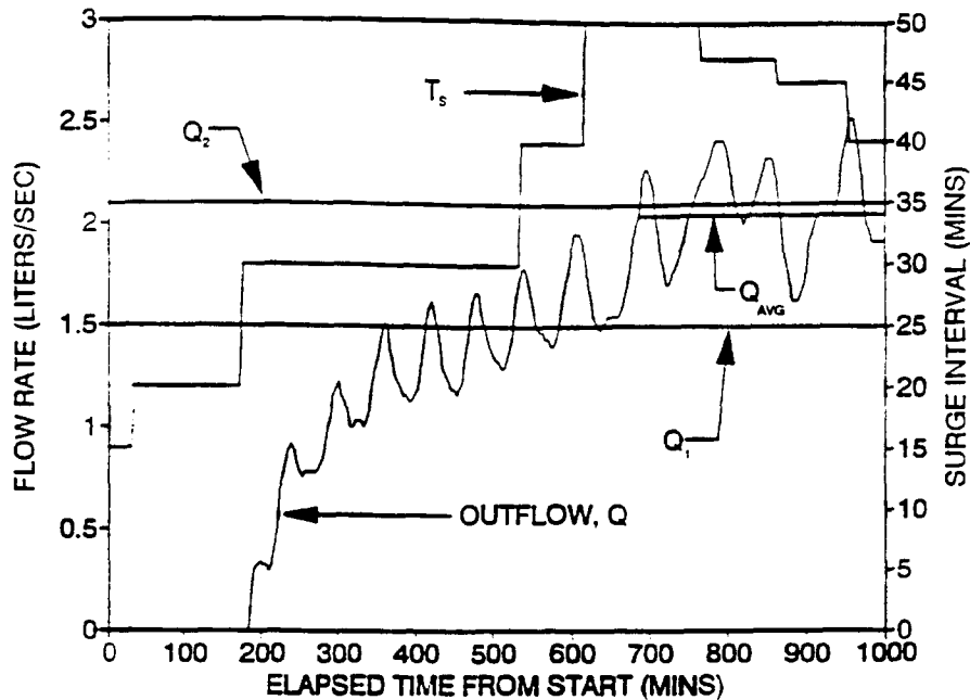
Figure 2. Output diagram which shows surge cycle intervals and actual and target runoff rates during cutback for an alfalfa field with a high water infiltration rate. (Diagramme des résultats illustrant les intervalles du cycle d'irrigation à impulsions ainsi que les taux d'écoulement actuels et de visée lors de la phase de réduction d'un champ d'alfafa avec un taux d'infiltration élevé.)
